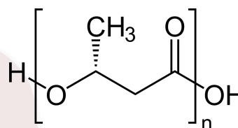
Figura 1: Polihidroxialcanoatos.
