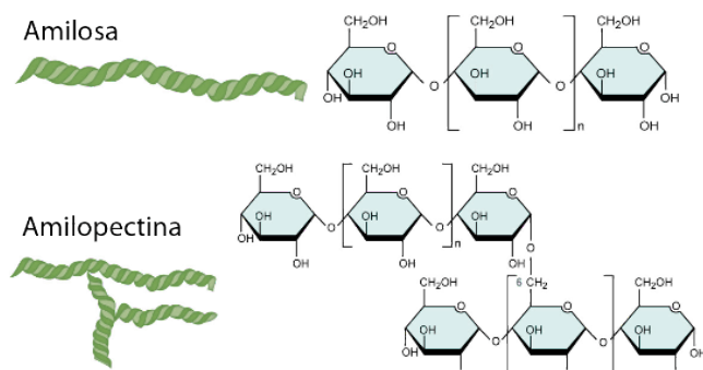
Figura 2: Estructura de la amilosa y amilopectina que forman el almidón
